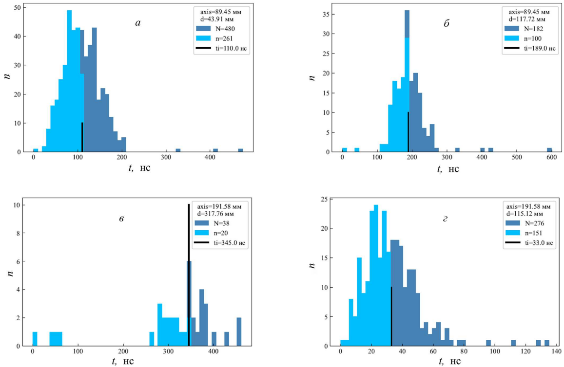
Рис. 7. примеры импульсов эксперимента в ФЭУ для произвольных клонов, при энергии 30 ПэВ. axis — расстояние от ближайшего к оси ливня ФЭУ до оси телескопа на мозаике; d — расстояние между данным ФЭУ и ФЭУ, ближайшим к оси ливня, на мозаике; N — число фотоэлектронов в ФЭУ
