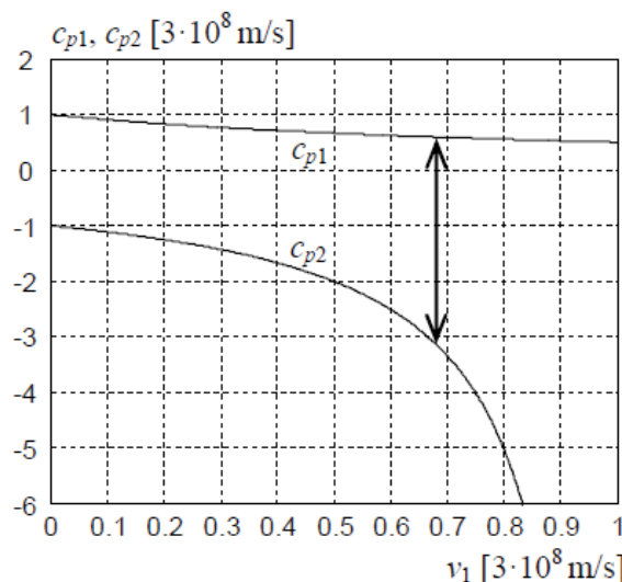
Рис. 3: Скорость света в инерциальной системе для v_1 \geq 0
